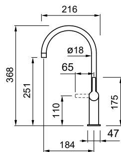
Einhandmischer mit schwenkbarem Auslauf Filtering tap with rotating spout
