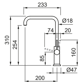
Einhandmischer mit schwenkbarem Auslauf Single-lever tap with swivel spout
