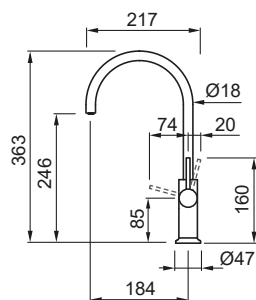
Einhandmischer mit schwenkbarem Auslauf Single-lever tap with swivel spout
