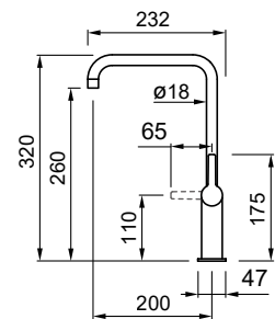
Einhandmischer mit schwenkbarem Auslauf Filtering tap with rotating spout
