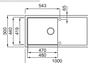
Ausschnittmaß Einbau von oben 980 x 480 mm Beckentiefe: 200 mm
